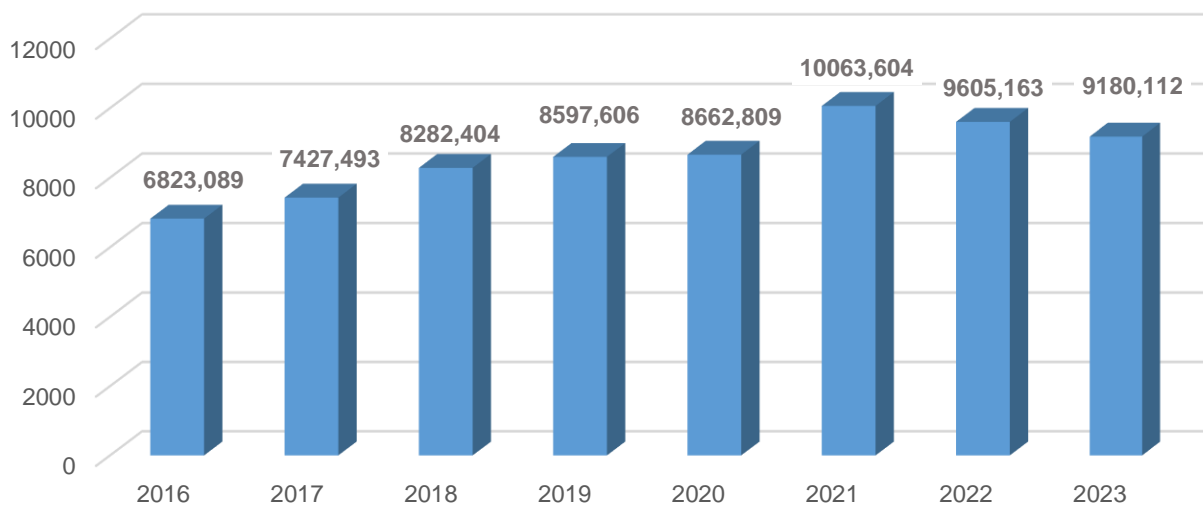
Elektros energijos sąnaudos MWh per metus
